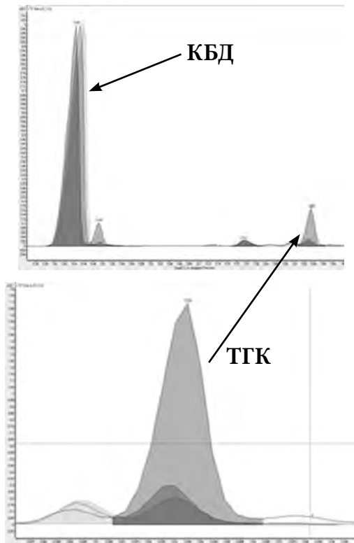
Рис. 2. Зображення порівняльного накладення хроматограм екстрактів, отриманих екстракцією однакових наважок досліджуваної рідини однією порцією (2 мл) таких розчинників: хлороформу – хроматограма зеленого кольору; діетилового ефіру – хроматограма фіолетового кольору; гексану – хроматограма червоного кольору)**
